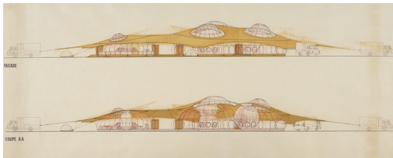
Antoine Stinco (A.J.S. Aérolande), Hall itinérant d'exposition d'objets de la vie quotidienne , 1967-1969 Élévation, façade et coupe AA, éch. 1:50 Dessin : encre, crayon de couleur, aquarelle et collage sur tirage papier, 69 x 169 cm Collection Frac Centre-Val de Loire, inv. 996 01 86 Photographie : François Lauginie
